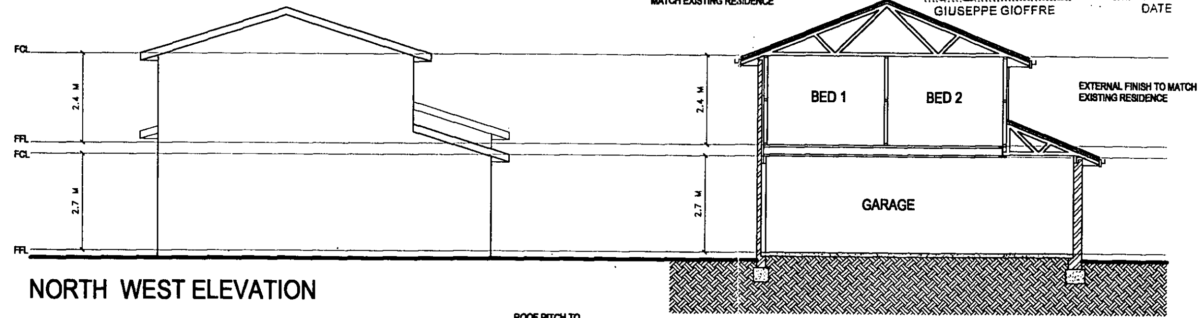
SECTION A-A
