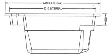
DEEP END ELEVATION
